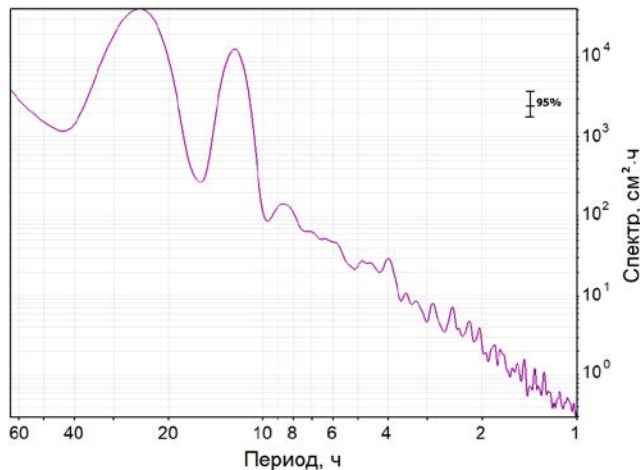
Р и с. 5. Рассчитанный по временному ряду продолжительностью 3,7 мес спектр приливных флуктуаций уровня по данным измерений прибора, расположенного вблизи м. Кастрикум Fig. 5. Spectrum of tidal fluctuations of the level at the instrument's location near Cape Castricum calculated from the 3.7-month-long time series
